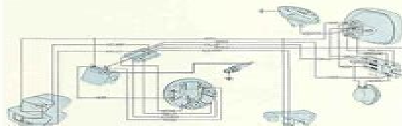
Fig. 24 - Installazione impianto elettrico sulla moto
