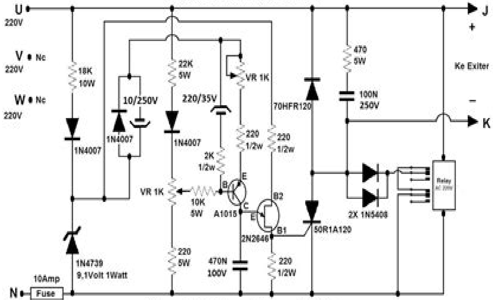
Skema AVR Universal 5 Sampai 500Kva
