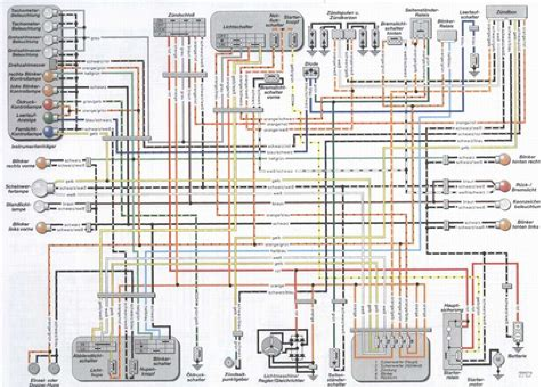
Schaltplan - GSF 600 (Europa-Modell)
