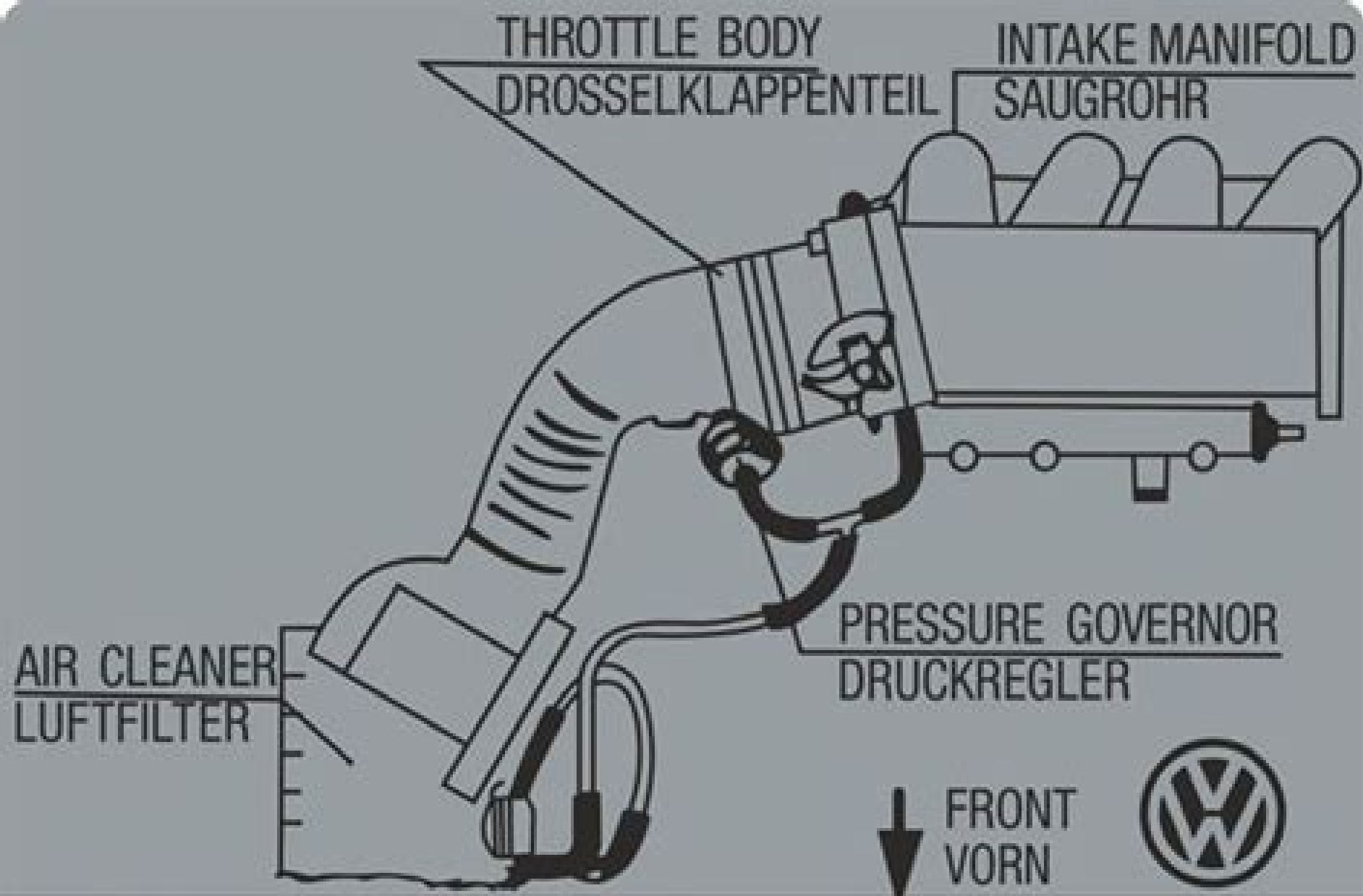
VACUUM HOSE ROUTING DIAGRAM ANORDNUNG DER UNTERDRUCKLEITUNGEN
