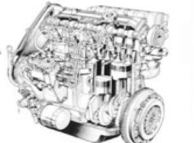
VISTA IN TRASPARENZA MOTORE 1000
