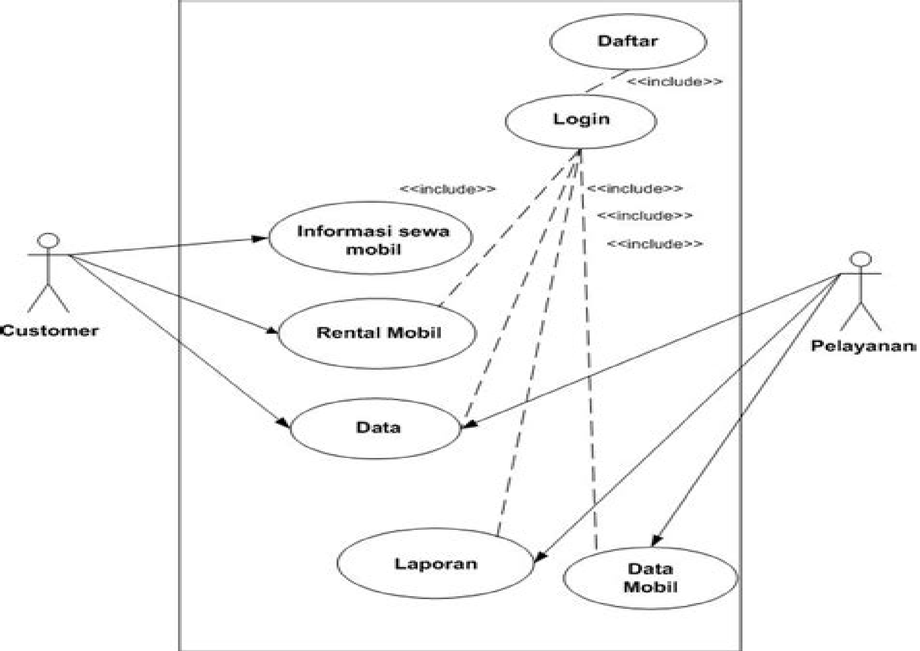
Gambar 2 Use Case Berjalan
