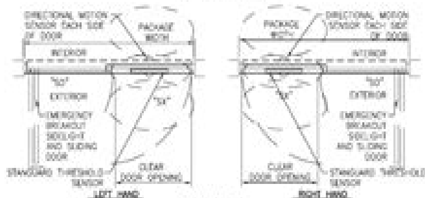
PLAN VIEW SCALE: 1/8" = 1'-0"
