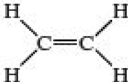
alkene
