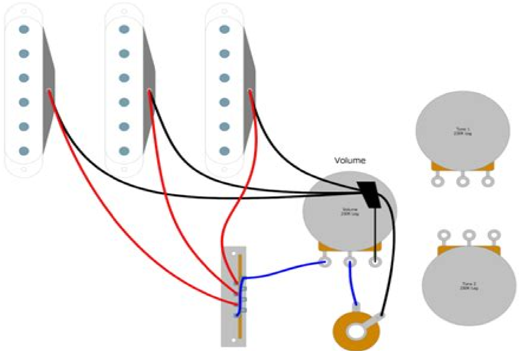
5 Way Switch
