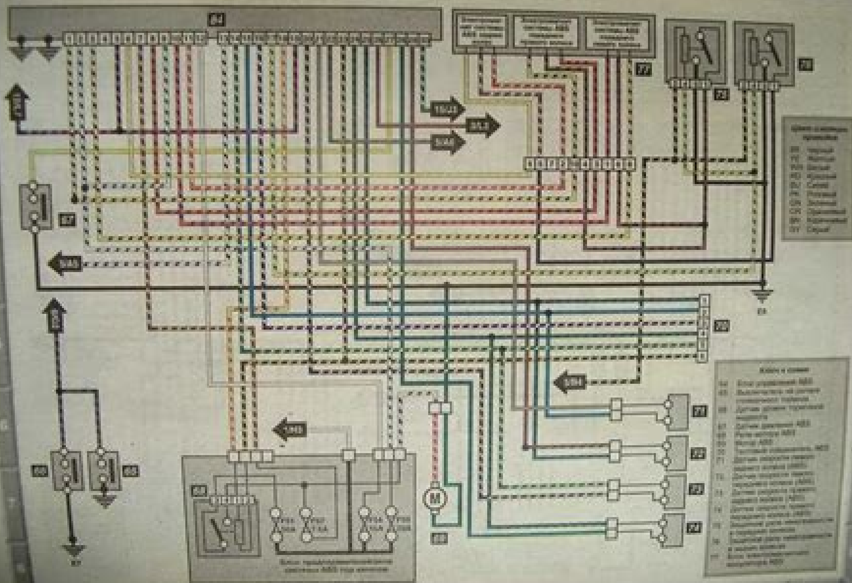
Схема 8: Типовой электрический план модели Civo - 8 из 15
