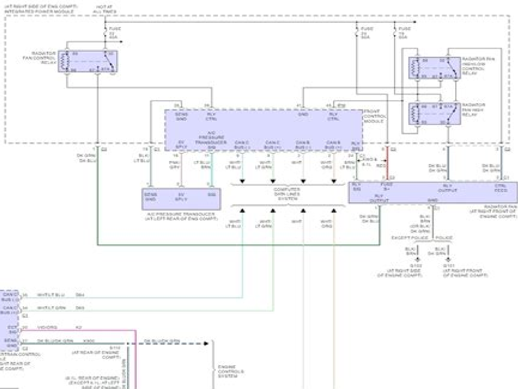
Fig 1: Cooling Fan Circuit
