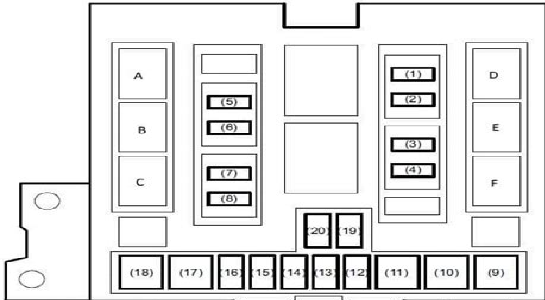
Блок реле № 1
