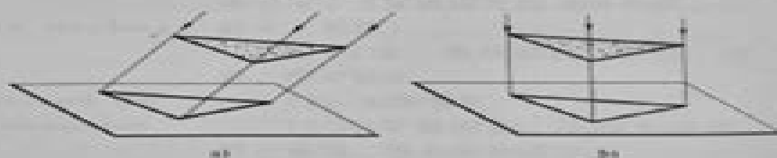
Fig. 2-2 Parallel projection 平行投影法 a) Oblique projection 斜投影法 b) Orthographic projection 正投影法
