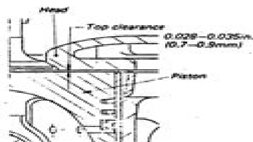
Fig. 21. Top Clearance
