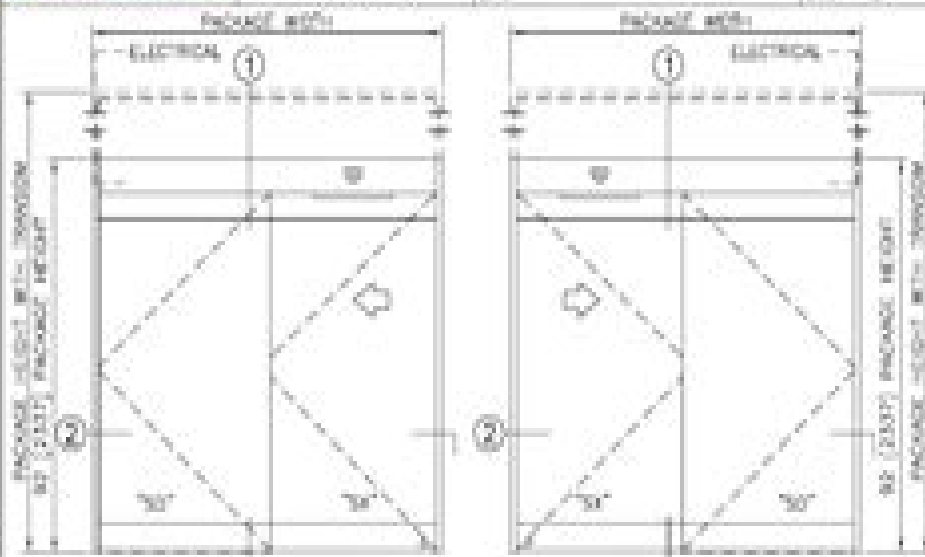
ELEVATION VIEW SCALE: 3/8" = 1'-0"
