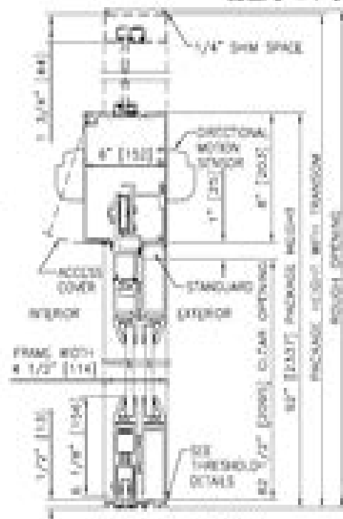
VERTICAL SECTION SCALE: 3/8" = 1'-0"
