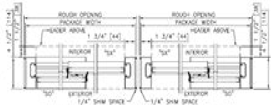
HORIZONTAL SECTION SCALE: 3/8" = 1'-0"
