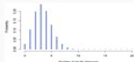
Binomial Distribution
