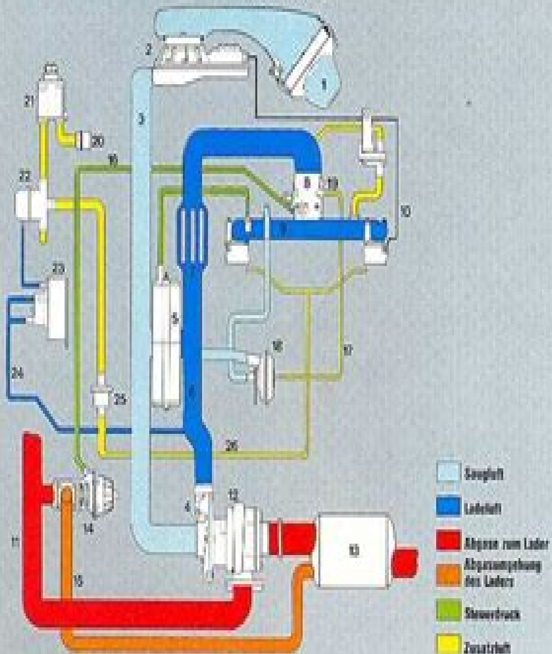
Funktionsschema
