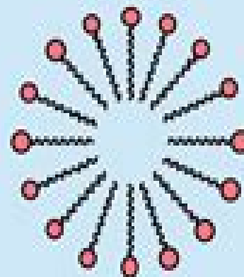
micelle
