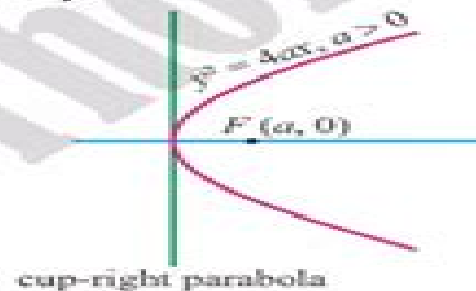
cup-right parabola
