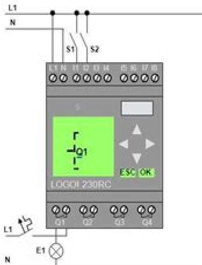
Logic module LOGO!
