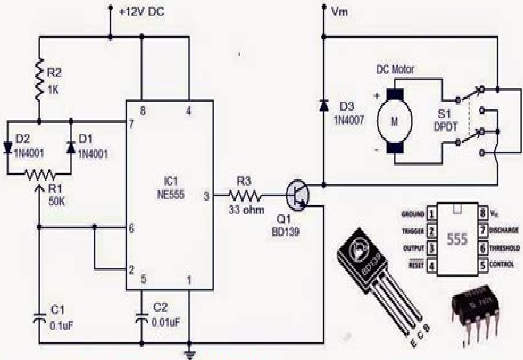
Rangkaian Pengendali Speed Motor DC
